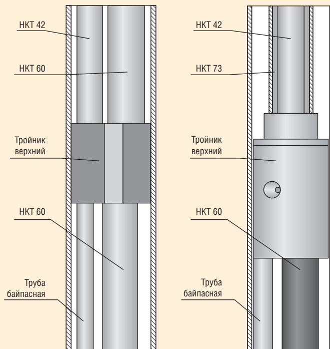
Рис. 2. Варианты исполнения напорных лифтов для компоновок ОРД
